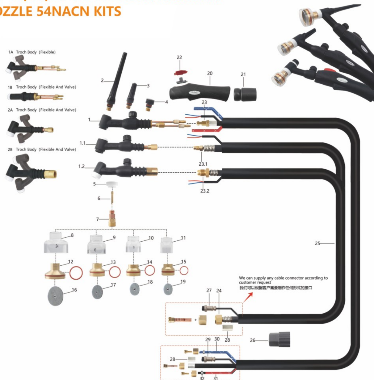
零件补/Parts
