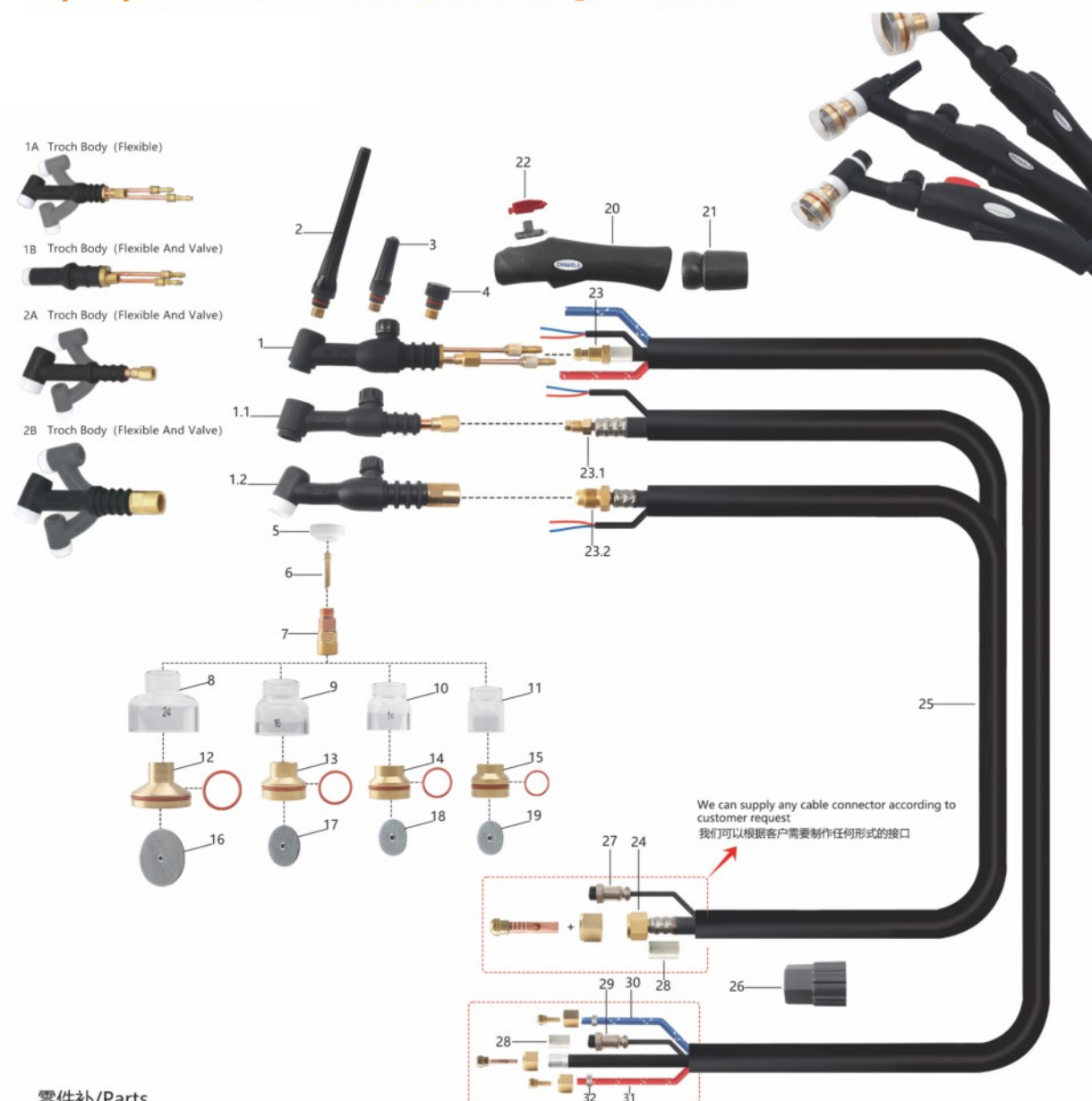
零件补/Parts
