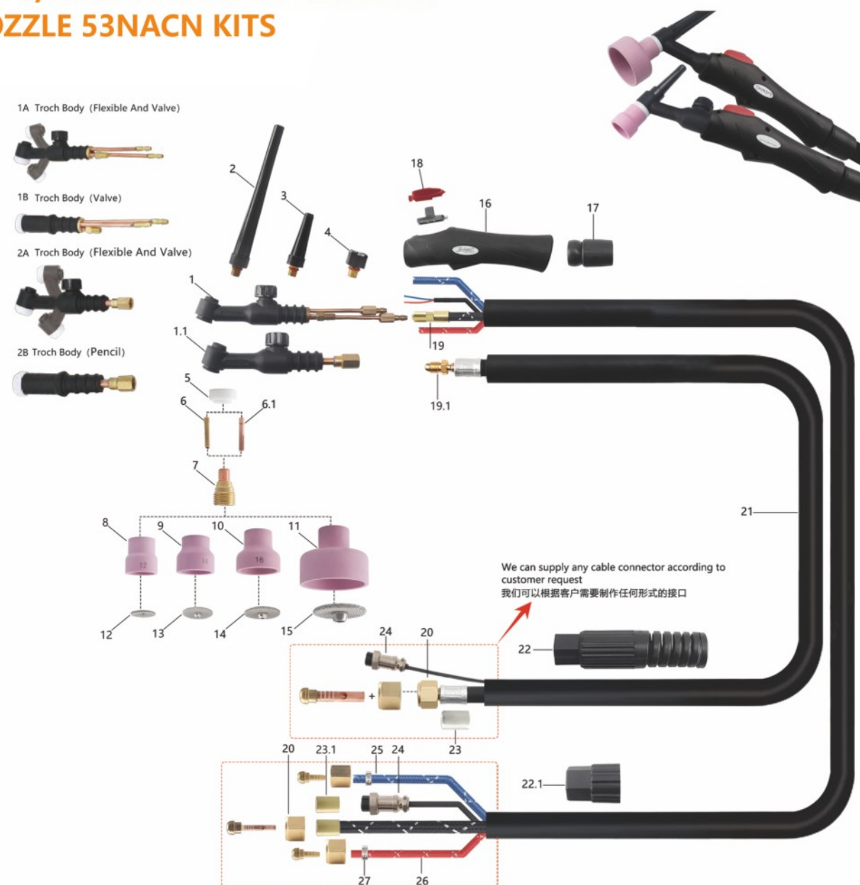
零件补/Parts
