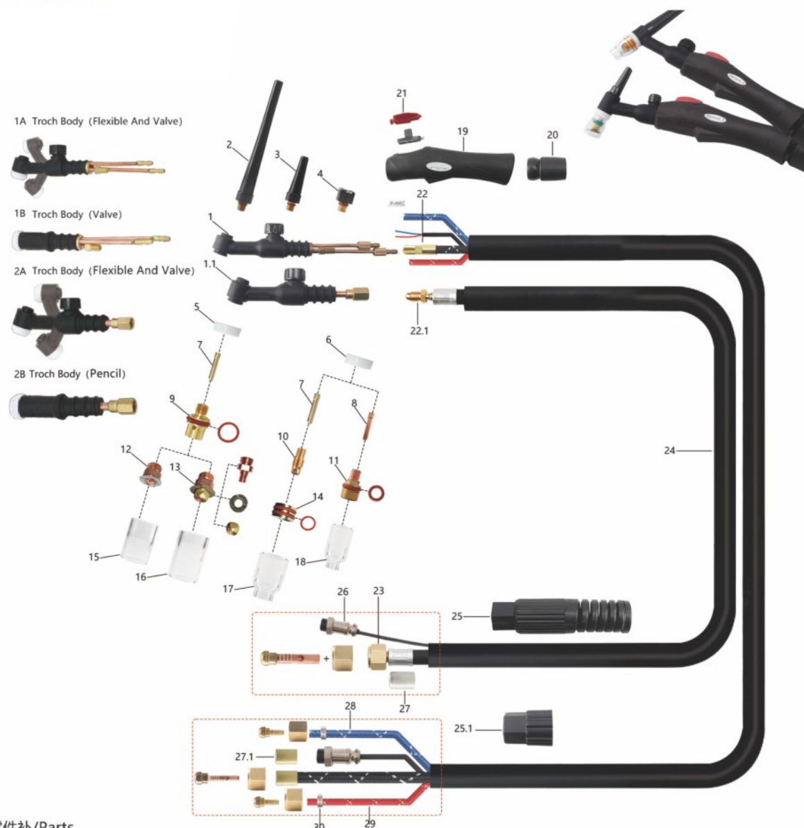
零件补/Parts
